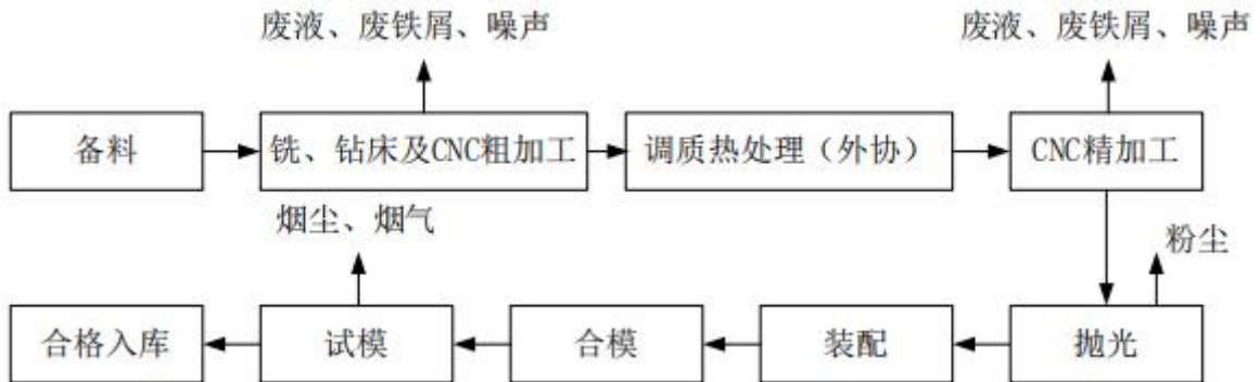
图 2-4 生产工艺流程图
