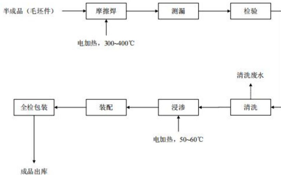
图 2-11 生产工艺流程图
