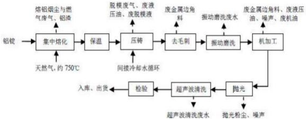
图 2-8 生产工艺流程图
