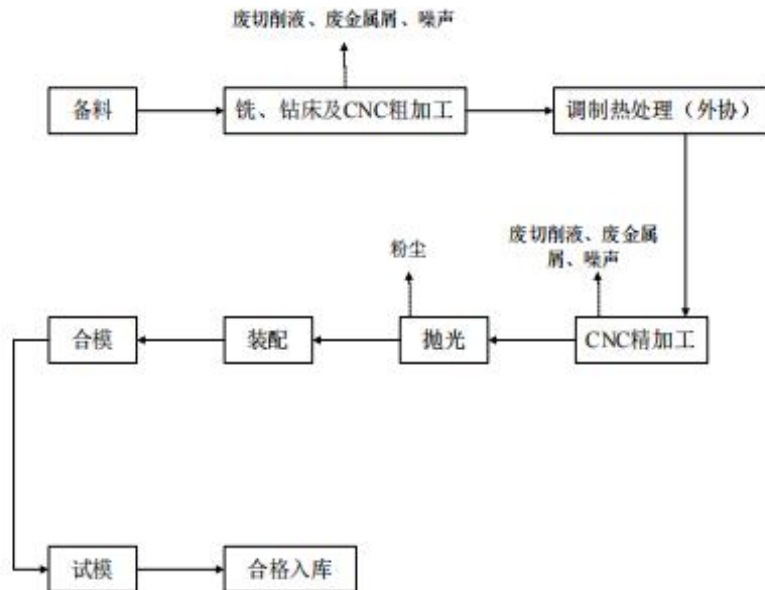
图 2-7 生产工艺流程图
