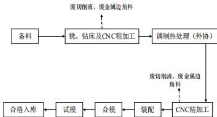
图 2-12 生产工艺流程图
