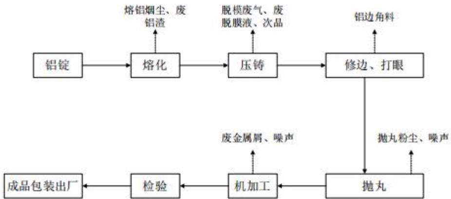
图 2-1 生产工艺流程图
