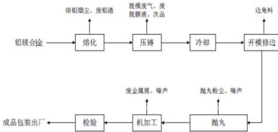
图 2-6 生产工艺流程图
