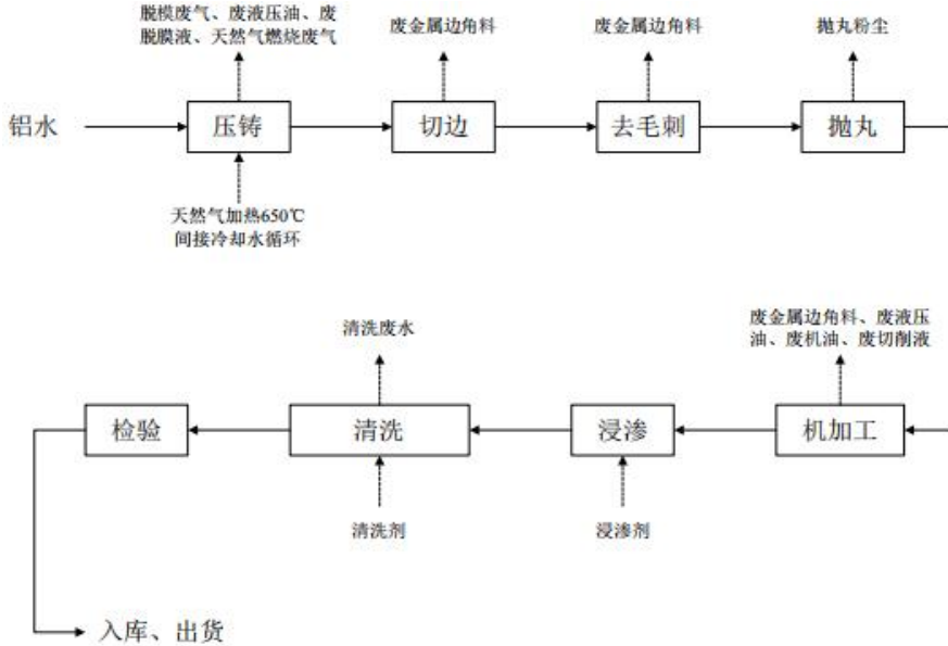
图 2-9 生产工艺流程图
