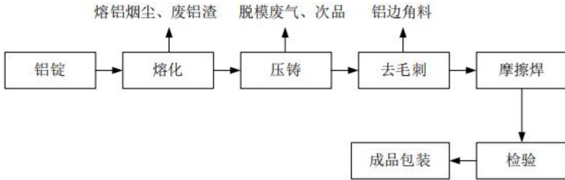
图 2-5 生产工艺流程图
